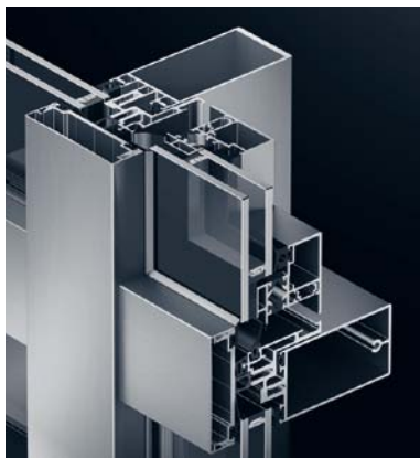
Schüco FW 50 + DK, unión en cruz Schüco FW 50 + DK façade joint
