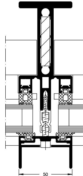
Schüco FW 50 + S, montante en forma de T, escala = 1:2 Schüco FW 50 + S, T-shaped mullion, scale = 1:2
