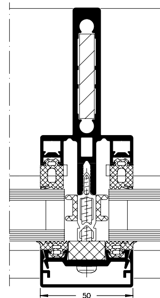
Schüco FW 50 + S.HI, montante en forma de I, escala = 1:2 Schüco FW 50 + S.HI, I-shaped mullion, scale = 1:2
